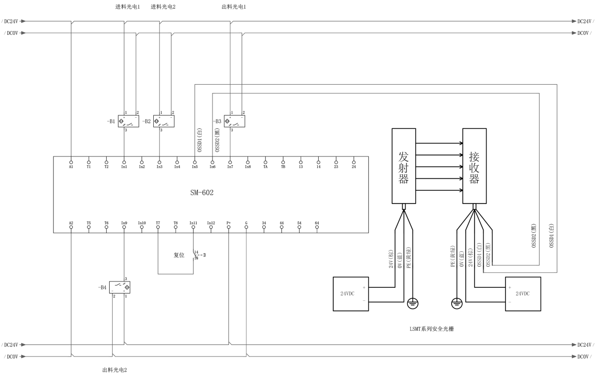
602双向平行进出料检测示意图
