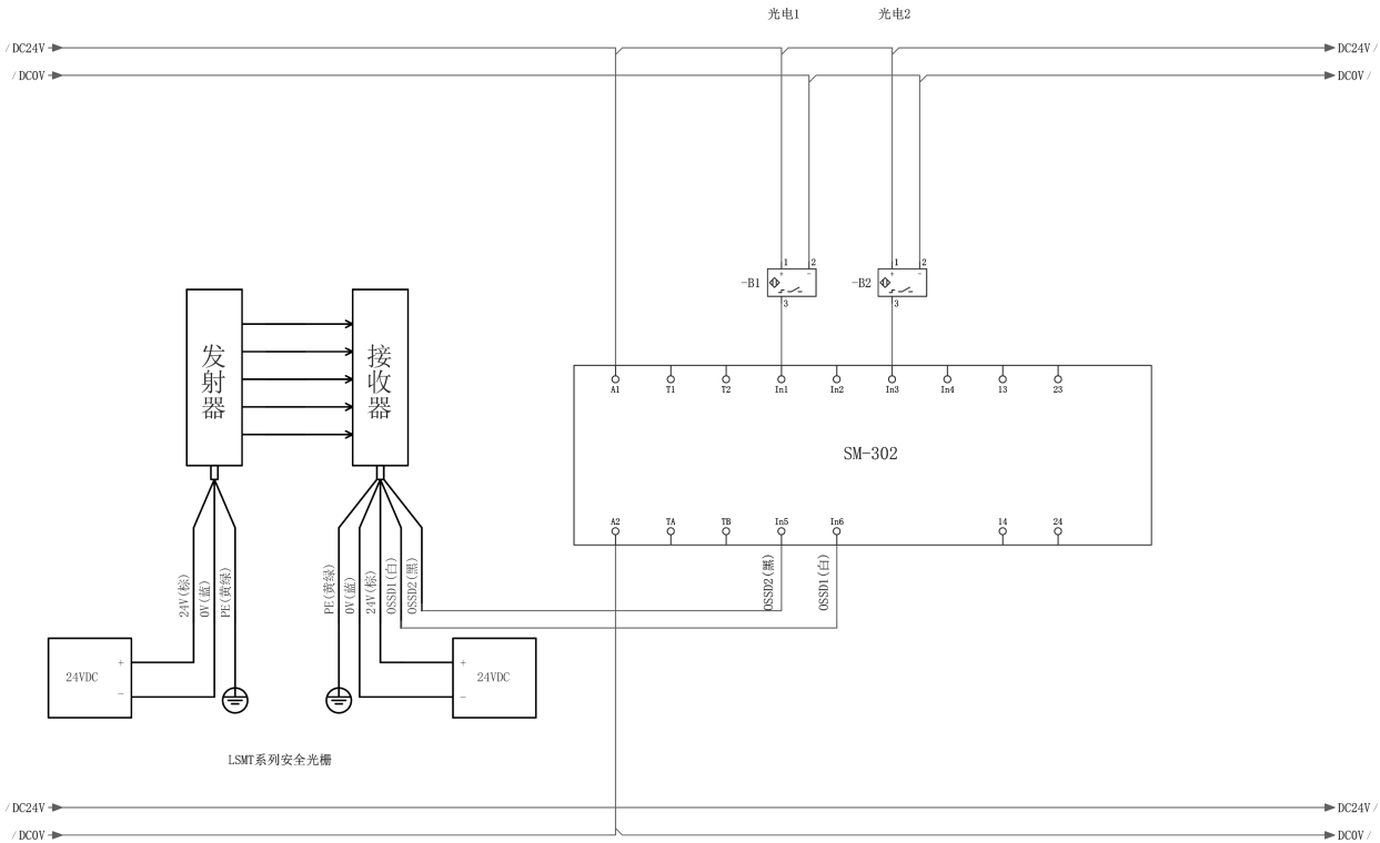
302交叉式进出料检测示意图
